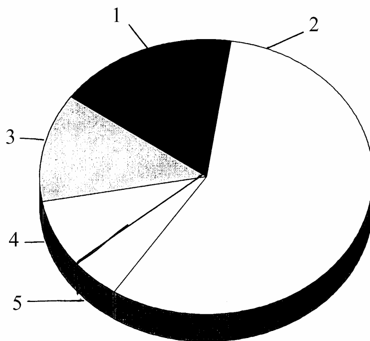
Fig. 1. Componența structurală a insecticidului biologic poliviral
